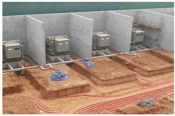
Steel & PVC Conduit
